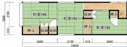
1階平面図
